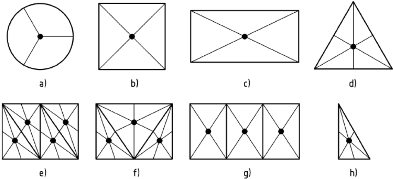
شکل ث-۱- مثال هایی از تعیین مرکز هندسی درپوش (ها) / قسمت (های) مشبک
