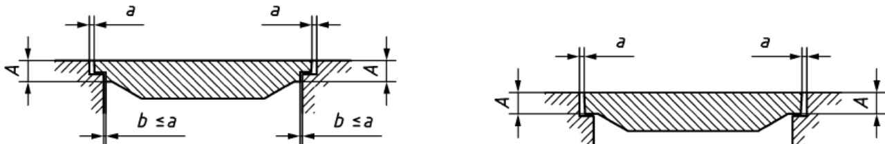
مثال ۲: A برای درپوش‌ها/قسمت‌های مشبک پله‌دار هنگامی که b \leq a
